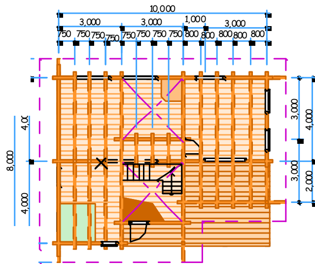
ロフト根太配置図
