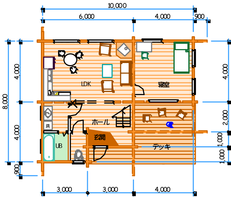
一階平面プラン 61.0㎡ (18.5坪)
