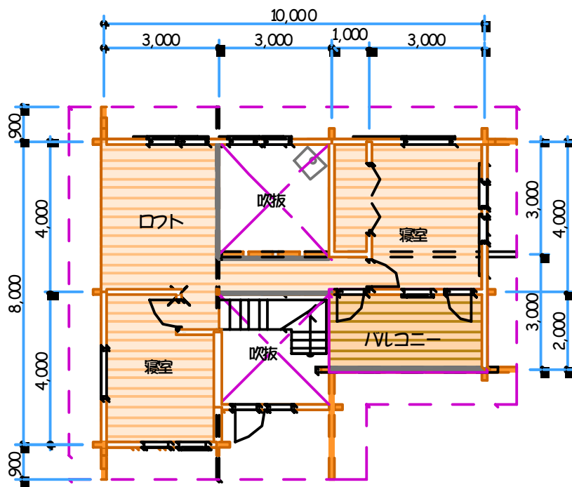
ロフト平面プラン 43.0㎡ (13.0坪)
