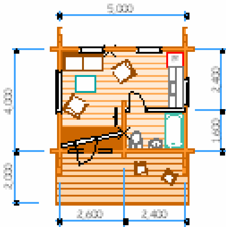
一階平面プラン 18.8㎡ (5.7坪)
