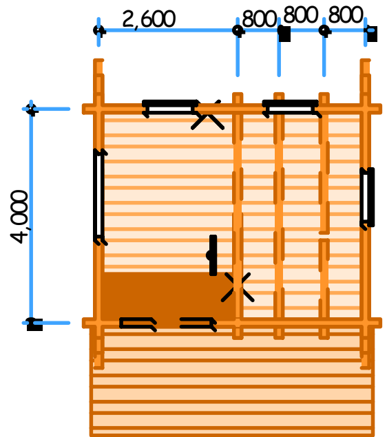
ロフト根太配置図
